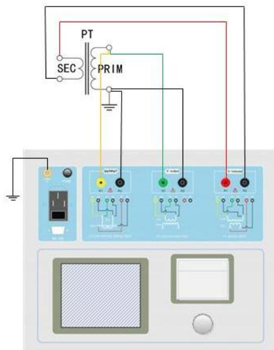
图 2.8 PT 变比试验接线方式
