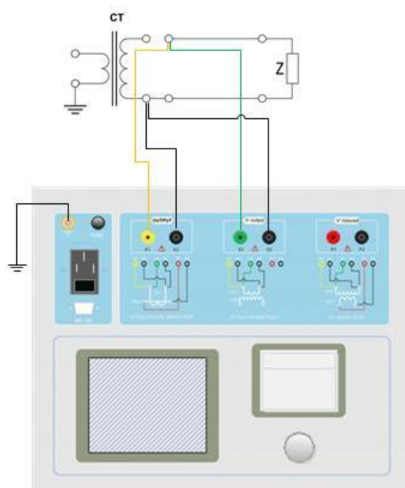
图2.2 CT负荷试验接线方式
