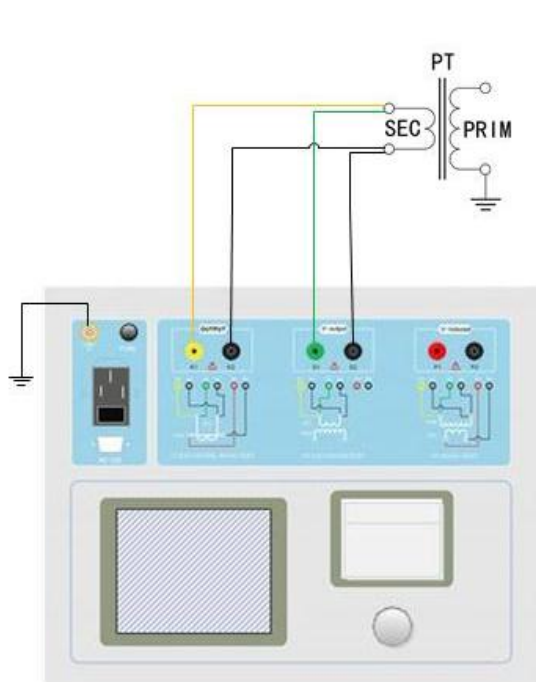
图 2.7 PT 直阻、励磁试验接线方式
