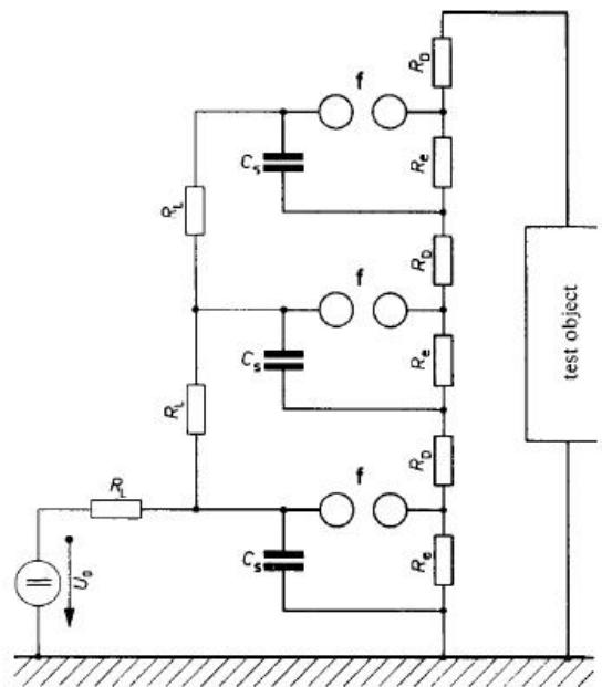
图 1 Marx回路（3级）示意图
