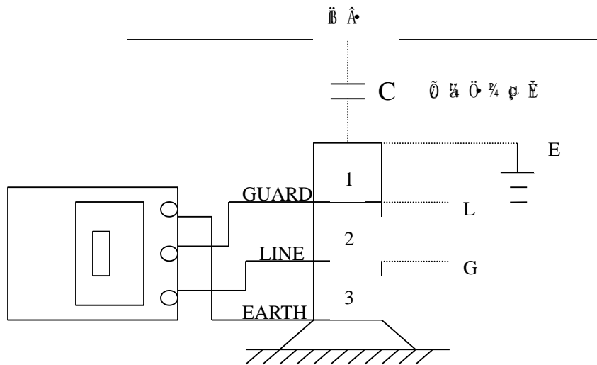
图 5 屏蔽端接法
